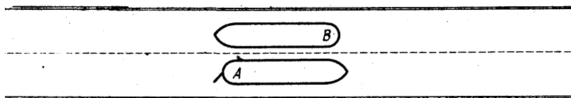
Рис. 89. Оба судна имеют тенденцию разворота влево. Судно А перекладывает руль вправо, чтобы остановить разворот, и этим самым создает опасную ситуацию •
