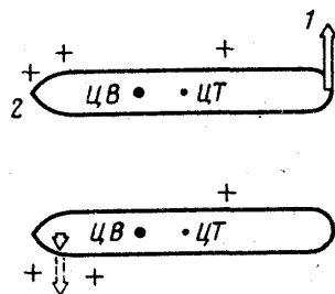
Рис. 36. Действие руля и носового подруливающего устройства, когда судно имеет ход: / — поперечная сила руля; 2 — боковое сопротивление
