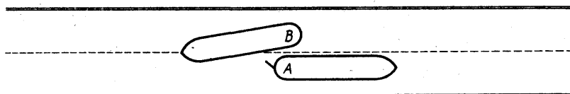
Рис. 90. Сейчас судно А испытывает присасывание судна В и должно положить руль на левый борт, чтобы избежать навала на берег. Нос судна В возвращается назад на центр канала; теперь корма будет возвращаться на ось канала в результате присасывания судна А
