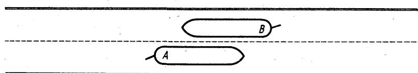
Рис. 87. Лево руля, чтобы корма прошла чисто. Носовые волны будут отталкивать форштевни судов в стороны
