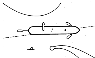
Рис. 83. Присасывание управляет судном:
