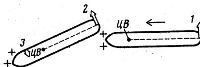
Рис. 10. Уменьшение усилия разворота, создаваемого рулем на судне, следующем передним ходом: 1 — начальный рычаг управления; 2 — рычаг управления; 3 — поперечное сопротивление
