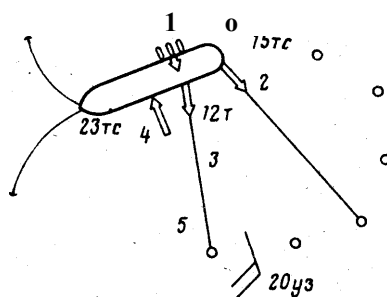
Рис. 26. Сила швартовной лебедки против силы ветра:
