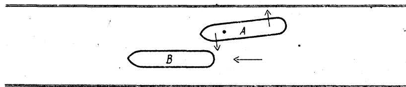
Рис. 96. Наиболее опасная ситуация, когда обгоняемое судно увеличивает скорость под влиянием попутного следа обгоняющего судна. Присасывание в носовой части обгоняемого судна и присасывание кормы вблизи берега образует сильную вращающую пару. Часто судно A необратимо подталкивается к корме судна B . Обгоняющее судно не испытывает особого влияния обгоняемого судна, оно должно бороться в основном с влиянием берегового эффекта
