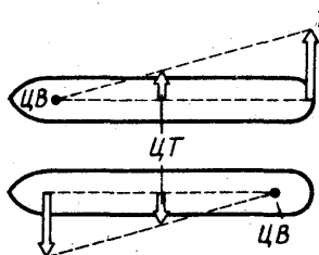
Рис. 34. Судно не имеет хода относительно воды:
