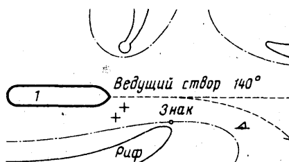
Рис. 81. Влияние носовой подушки в Восточном проливе Аруба: 1 — судно дедвейтом 85 тыс. т, осадка на ровном киле 41 фут, глубина 45 футов.
