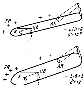
Рис. 121. Поперечное сопротивление позади ЦВ ограничивает угол дрейфа:
