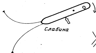
Рис. 67. Воздействие ветра, когда сохраняется слабина левой якорной цепи
