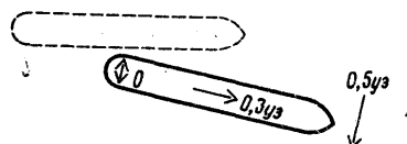
Рис. 109. Использование машины и руля, когда судно имеет поперечное движение
