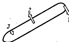
Рис. 17. Удержание на курсе при перекладке руля на другой борт: 1 — поперечная сила от действия руля; 2 — направление поперечной инерции движения; 3 — боковое сопротивление
