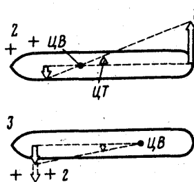
Рис. 35. Судно движется вперед с очень малой скоростью:
