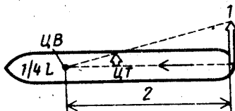
Рис. 14. Влияние поперечной силы руля на ход:
