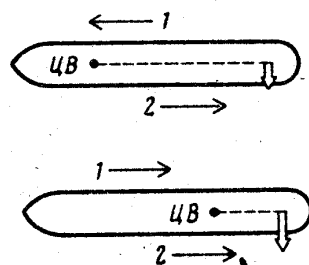
Рис. 18. Поперечная сила и ЦВ: / — движение судна; 2 — машина работает назад
