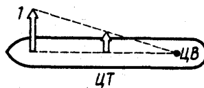
Рис. 33. Действие поперечного упора:
