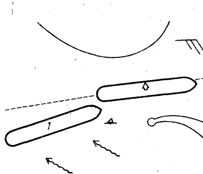
Рис. 59. Поперечный снос танкера в балласте: 1 — судно дедвейтом 85 тыс. т; T_n = 16 футов; T_k = 26 футов
