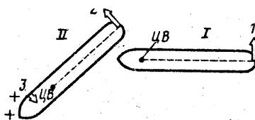
Рис. 9. Уменьшение разворачивающего плеча руля из-за движения вперед: / — судно не имеет хода относительно воды; // — судно дало ход вперед; / — Начальный рычаг управления; 2 — рычаг управления; 3 — поперечное сопротивление
