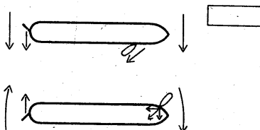
Рис. 43. Буксир толкает или буксирует под углом
