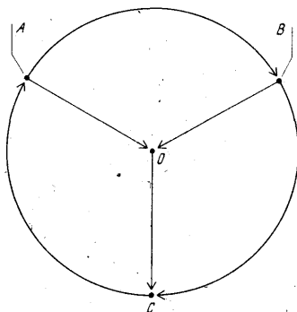
Рис. 122. Зависимость между действием силы руля, углом дрейфа, поперечным сопротивлением и ЦВ
