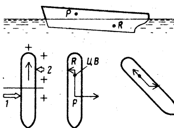
Рис. 7. Действие ветра на судно на заднем ходу: 1 — ветер; 2 — поперечное сопротивление
