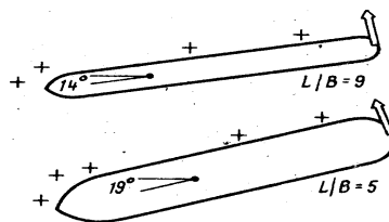
Рис. 15. Влияние ширины судна на ЦВ и угол дрейфа
