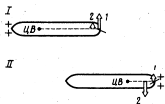
Рис. 11. Поперечная сила от действия руля и поперечный упор:
