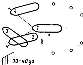
Рис. 75. Сильный ветер в левую скулу при отходе от СВМ
