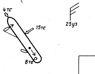
Рис. 48. Ветер 30° по носу
