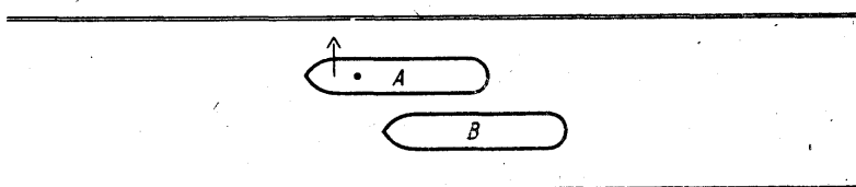
Рис. 93. На этой стадии обгоняемое судно А уже испытывает влияние обгоняющего судна В. Носовая волна от судна В придает ускорение судну А и в то же самое время отталкивает корму в сторону. Этот эффект будет усугублять эффект присасывания кормы
