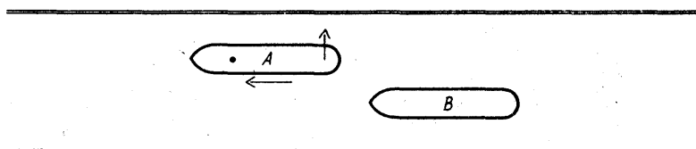
Рис. 93. На этой стадии обгоняемое судно А уже испытывает влияние обгоняющего судна В. Носовая волна от судна В придает ускорение судну А и в то же самое время отталкивает корму в сторону. Этот эффект будет усугублять эффект присасывания кормы
