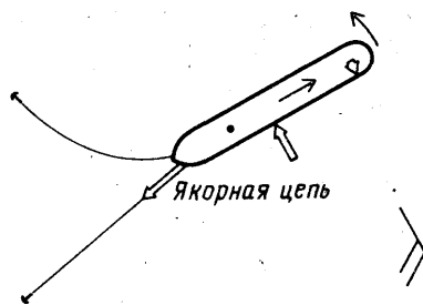
Рис. 68. Воздействие ветра, когда левая якорная цепь набита
