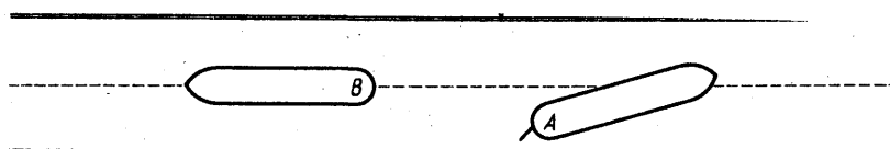
Рис. 92. С помощью перекладки руля право на борт судно А не смогло остановить рыскание, вызванное присасыванием. Судно В использовало Взаимодействие судов с пользой для себя
