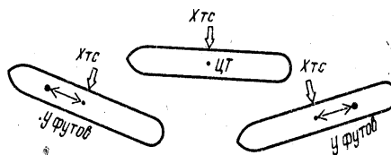
Рис. 114. Действие поперечной силы при продольном движении
