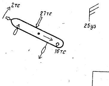
Рис. 47. Ветер 60^\circ по носу
