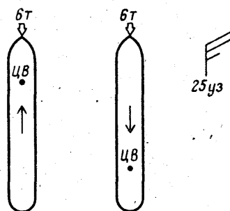
Рис. 19. Действие ветра по носу на танкер дедвейтом 70 тыс. т в балласте
