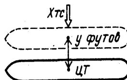
Рис. 113. Действие поперечной силы на судно на ровном киле и не имеющее хода относительно воды
