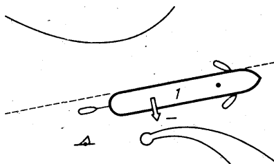
Рис. 84. • Присасывание нежелательного борта:
