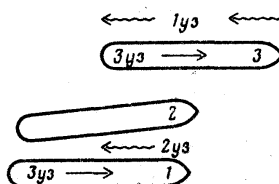
Рис. 57. Увеличение скорости судна относительно грунта при уменьшении скорости встречного течения помощь лага, дающего скорость относительно грунта и относительно воды.
