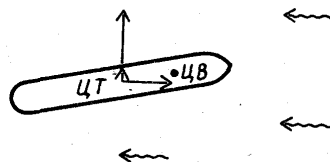
Рис. 55. Боковое смещение и боковая инерция
