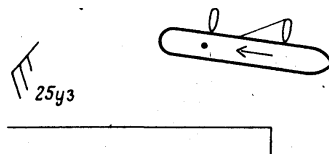
Рис. 99. Постановка к причалу кормой вперед при отжимном ветре
