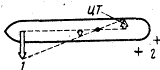
Рис. 37. Действие носового подруливающего устройства на заднем ходу: / — сила НПУ; 2 — боковое сопротивление
