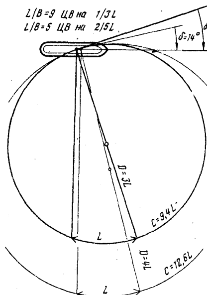
Рис. 123. Теоретические кривые циркуляции и угла дрейфа для различных отношений L/B ной циркуляции.
