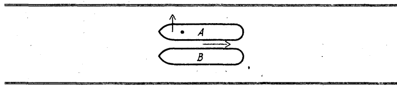
Рис. 95. Две носовые волны отталкивают носовые части судна в стороны. Взаимное присасывание сводит кормы вместе и в то же время скорость судна A значительно снижается. Судно B разворачивается в сторону берега при уменьшившейся скорости и этому не нужно противодействовать, поскольку это может создать для него опасную ситуацию
